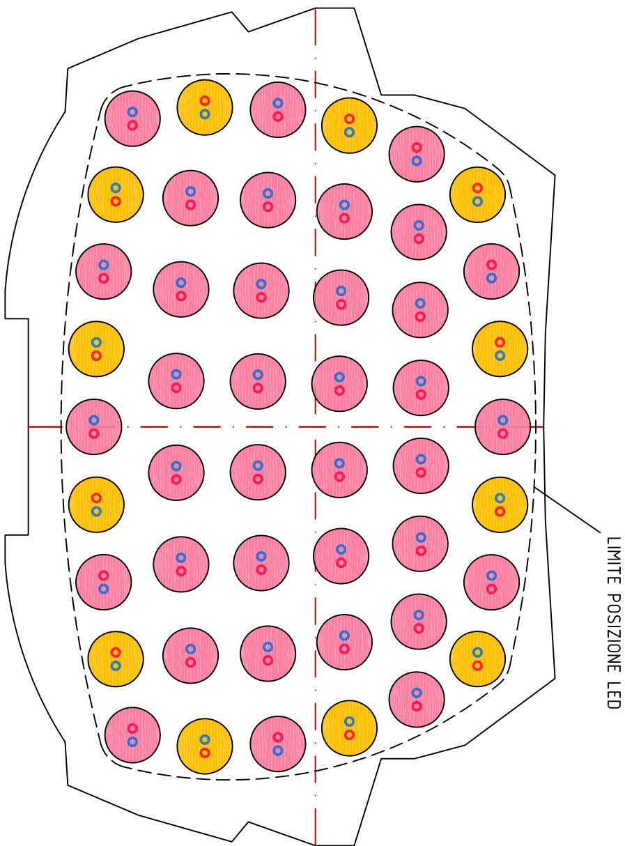
LED FISSATI SENZA INCLINAZIONE
