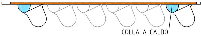
LED FISSATI CON INCLINAZIONE CREATA MEDIANTE COLLA A CALDO
