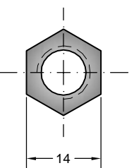
TESTA ESAGONALE
