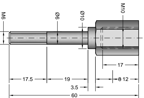
TESTA ESAGONALE
