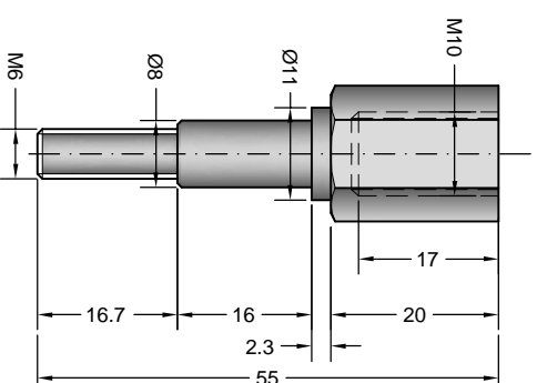
TESTA ESAGONALE
